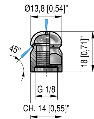
ST4 STURATUBO FISSI - 4 FORI ST4 DRAIN CLEANING NOZZLE - 4 HOLES
